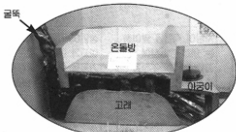
온돌의 구조
